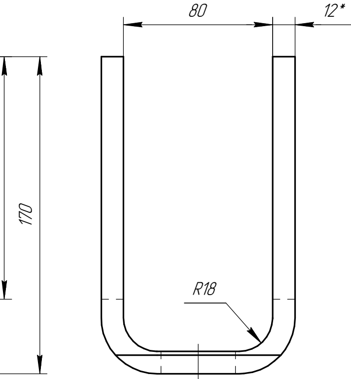
Дет. поз. 4 (1:2)
