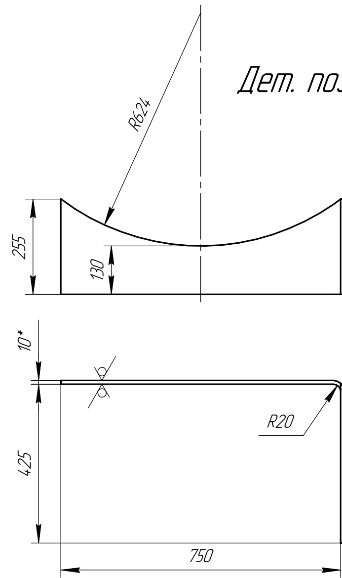
Дет. поз. 4 (1:2)
